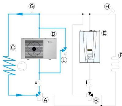
Hűtés hőszivattyúról
