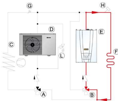
Fűtés csak kazánról
