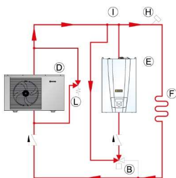
Fűtés hőszivattyúról, kazán integrálásával
