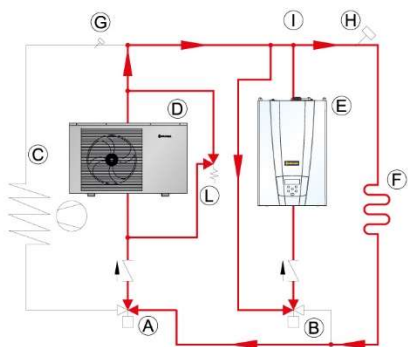
Fűtés hőszivattyúról, kazán integrálásával
