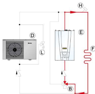
Fűtés csak kazánról
