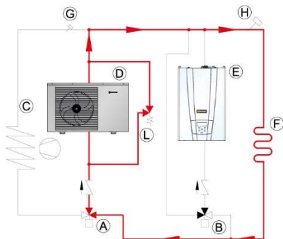
Fűtés hőszivattyúról
