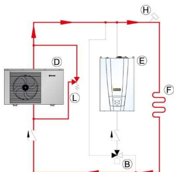
Fűtés hőszivattyúról
