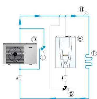
Hűtés hőszivattyúról
