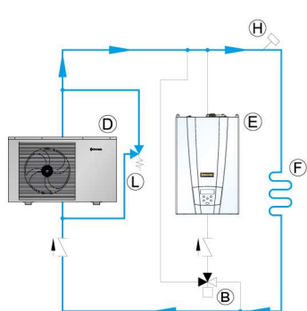
Hűtés hőszivattyúról
