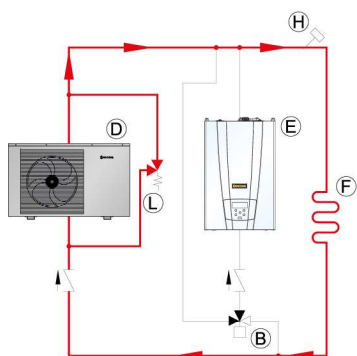
Fűtés hőszivattyúról
