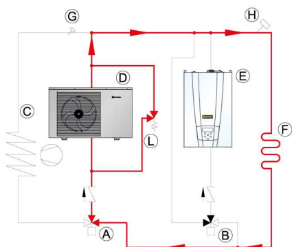
Fűtés hőszivattyúról
