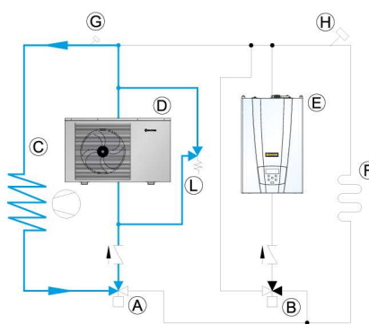
Hűtés hőszivattyúról
