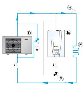
Hűtés hőszivattyúról
