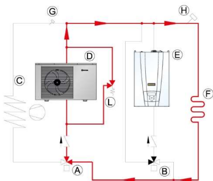
Fűtés hőszivattyúról
