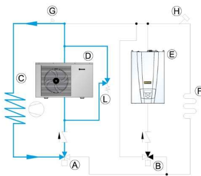
Hűtés hőszivattyúról
